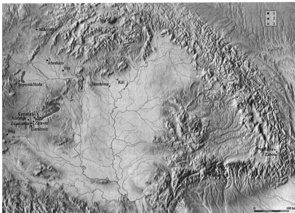
7. kép: A petőfalvai és zabolai temető „székelyeinek” genetikai kapcsolatai (Benkő, 2010. 231. p. 4. ábra nyomán)
